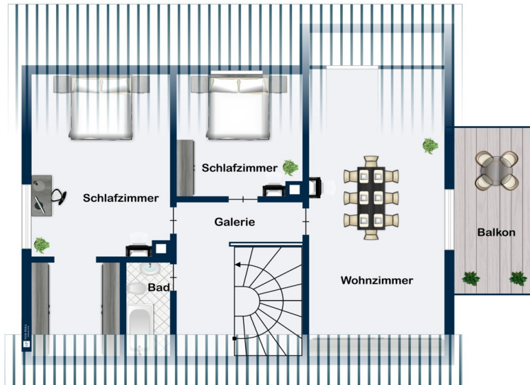
Dachgeschoss
