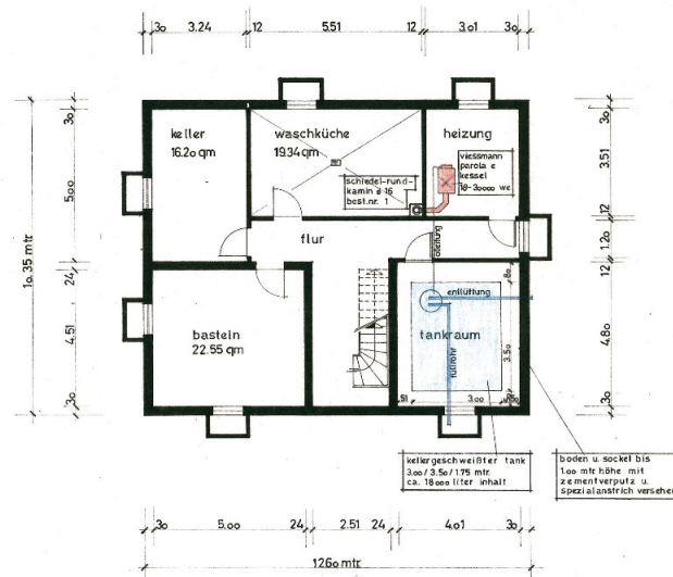
kellergeschoss
