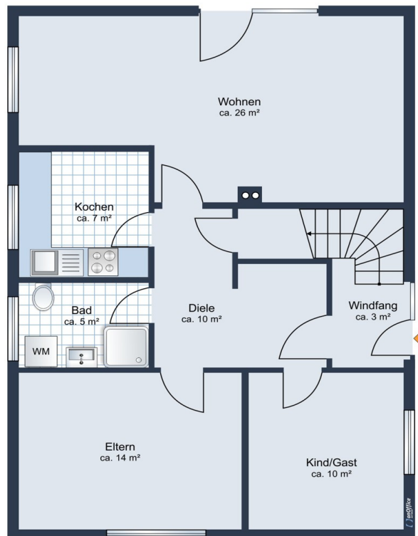
Erdgeschoss
