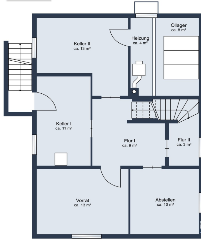
Kellergeschoss
