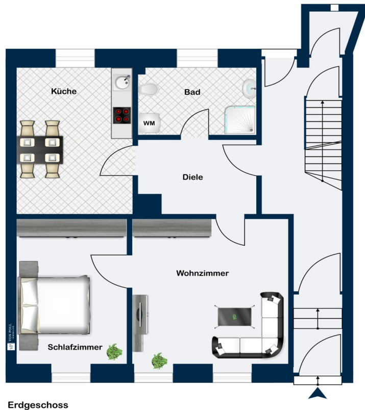
Erdgeschoss
