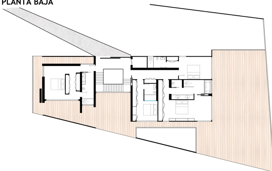
PLANTA BAJA
