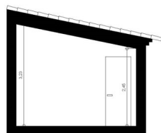
SECCIÓN A-A:
