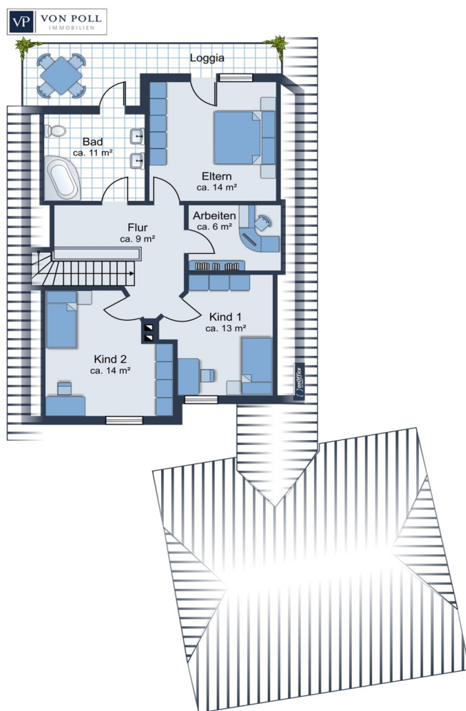
Obergeschoss
