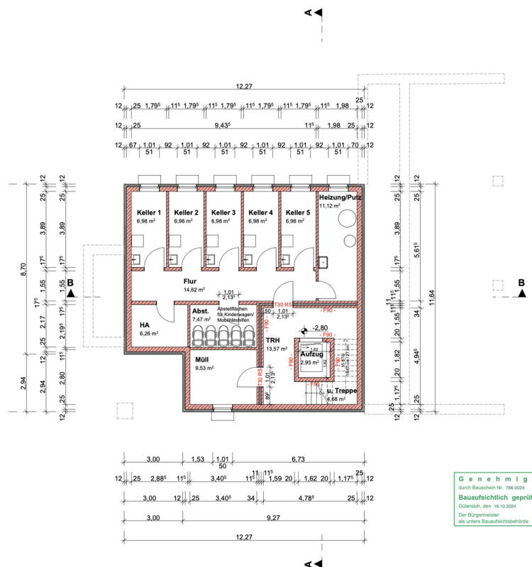
GRUNDRISS UG
