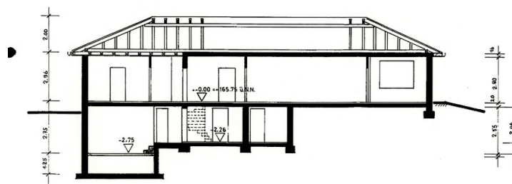
SCHNITT A-A
