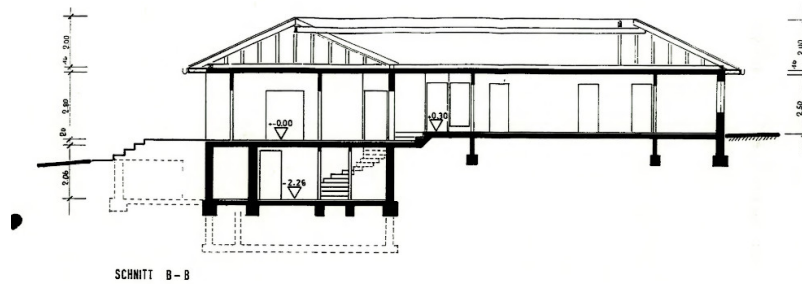
SCHNITT B-B
