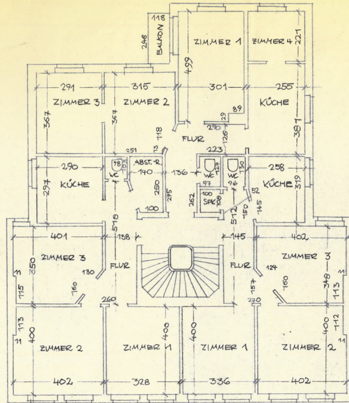
1. - 3. OBERGESCHOSS
