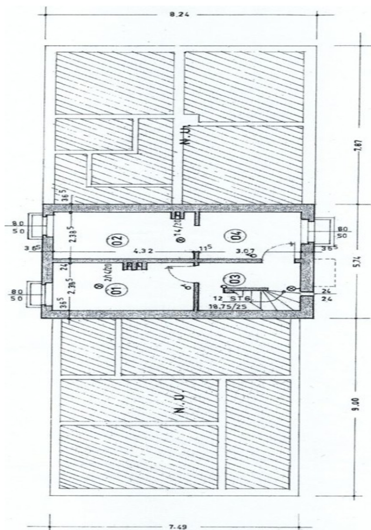
KELLERGESCHOSS GRUNDRISS
