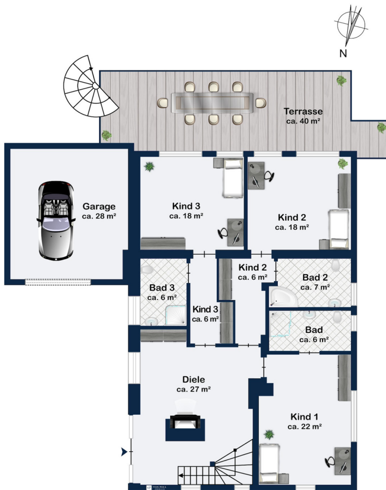
Erdgeschoss
