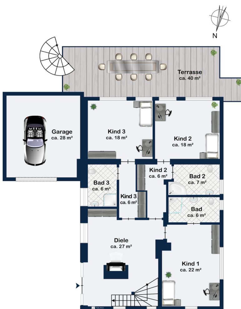
Erdgeschoss
