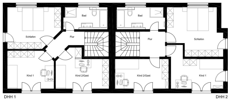
DHH 1 Grundriss OG
