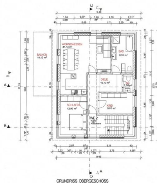
GRUNDRISS OBERGESCHOSS
