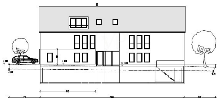
Ansicht Nord
