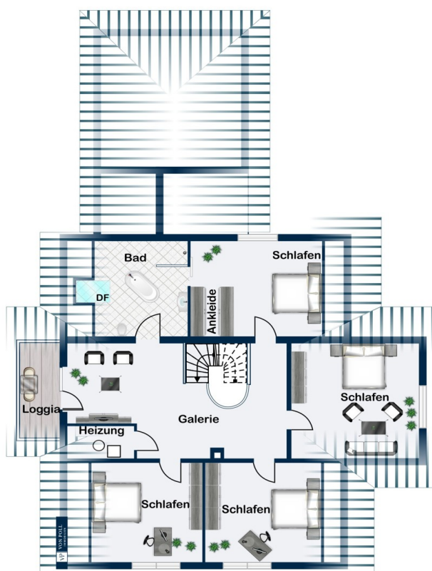
Dachgeschoss
