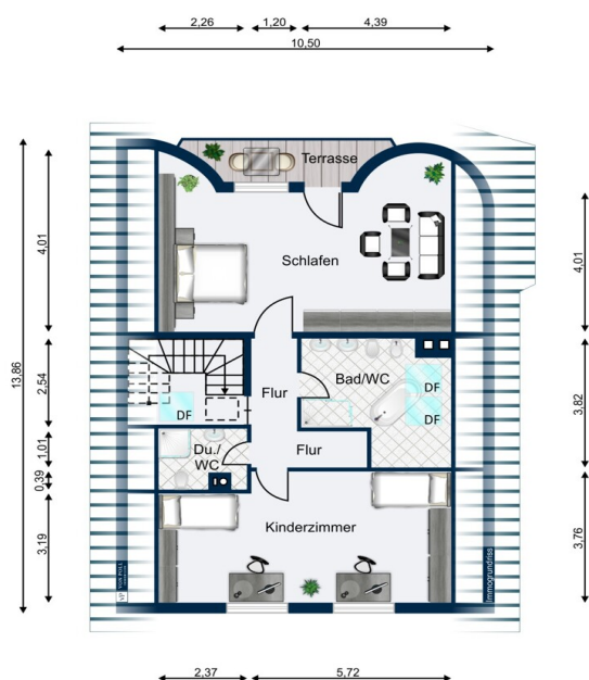
Dachgeschoss
