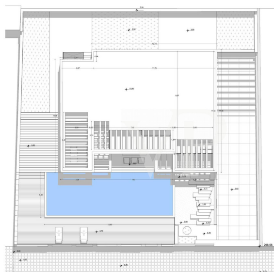
PLANTA DE TELHADO
