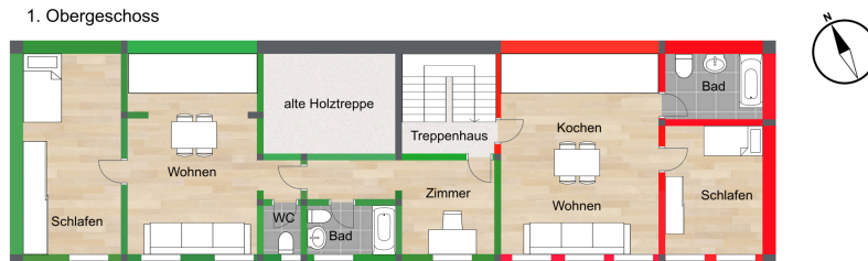
1. Obergeschoss
